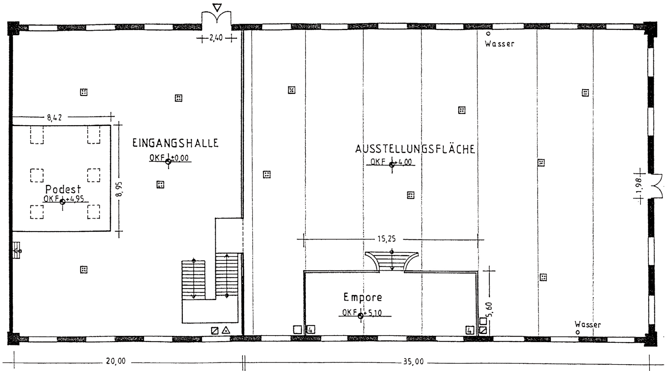
Grundriß M 1: 200
